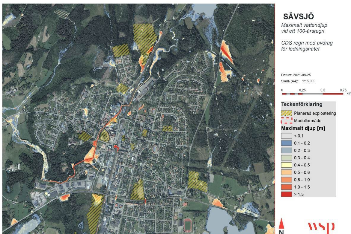
Bild 1. Maximala vattendjup vid ett klimatanpassat 100-årsregn, Sävsjö tätort.
