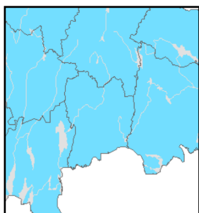
Figur 14. Förändring av nederbörd på enbart vår, beräknat till 2098. Länsstyrelsen i Jönköpings län 2017.
